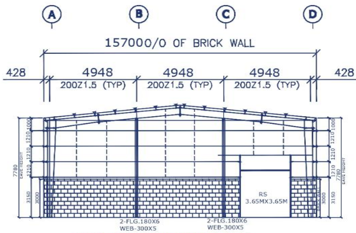
END WALL FRAMING ELE @ GL -1
